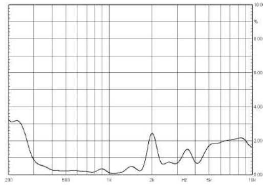
Distortion (THD< 3% 1W、1m、400Hz-8kHz)
